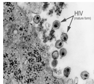
ヒト免疫不全ウイルス CDC
